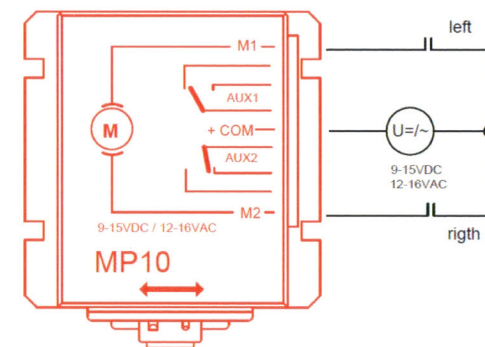
3 wire schematic MP1, MP4, MP8, MP10
